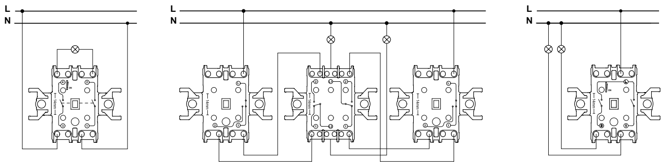
Двуполюсен ключ
